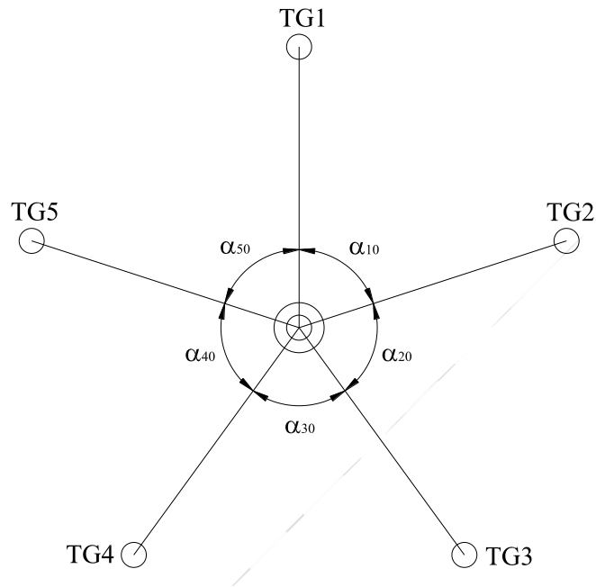
Hình 2. Sơ đồ bố trí hệ thống kiểm tra góc bằng
