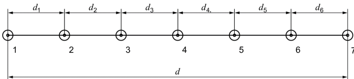
Hình 4. Đường chuẩn và các khoảng cách chuẩn
