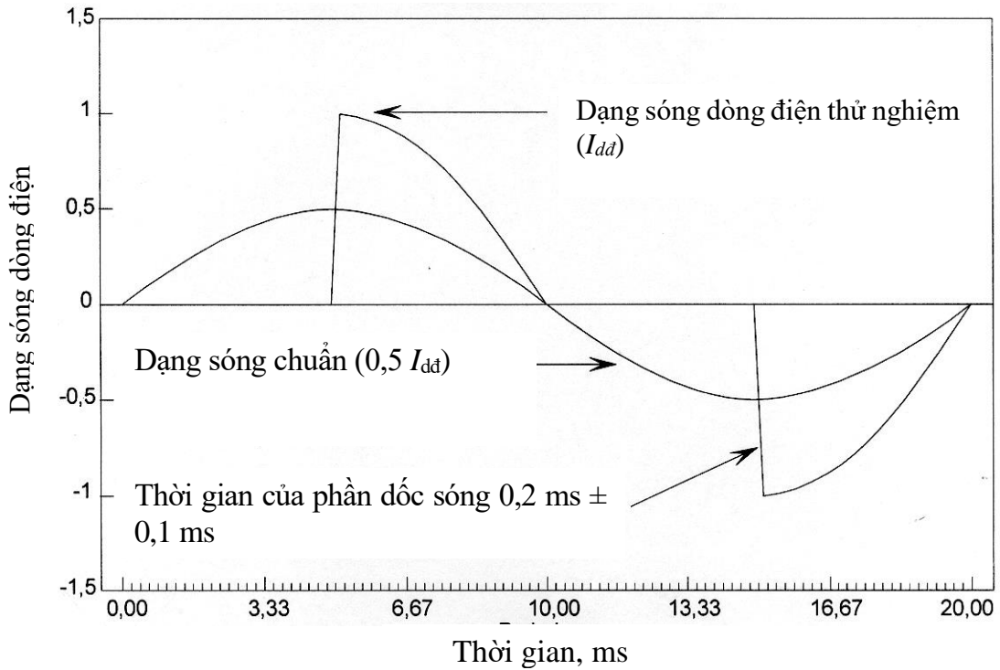
Hình 2. Dạng sóng hài bậc lẻ trong mạch dòng điện
