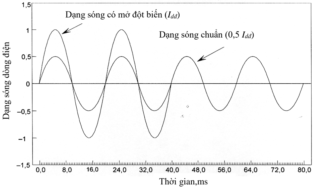
Hình 1. Dạng sóng hài phụ trong mạch dòng điện
